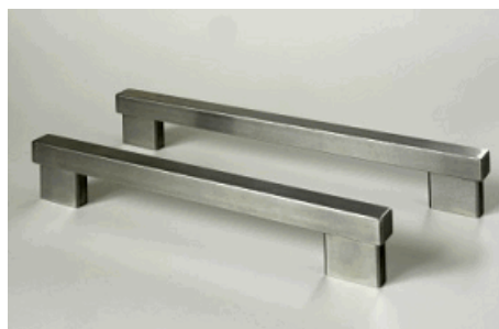
Úchytky broušená nerez. ocel,rozteč 128mm(2)
