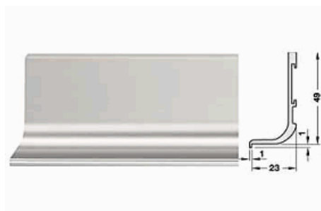
126.37.000 Zapuštěná úchytky alu.ststc.2500mm
