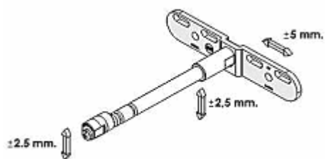
skrytá policová konsole 175 mm zinek / trn T/
