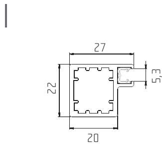
Průřez
