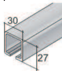
profil S80
